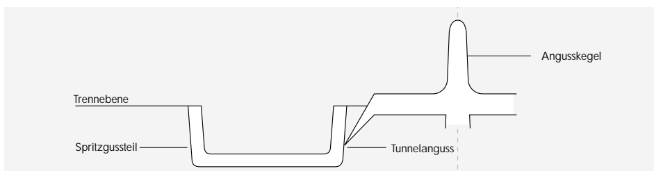
Abbildung 6: Tunnelanguss.
